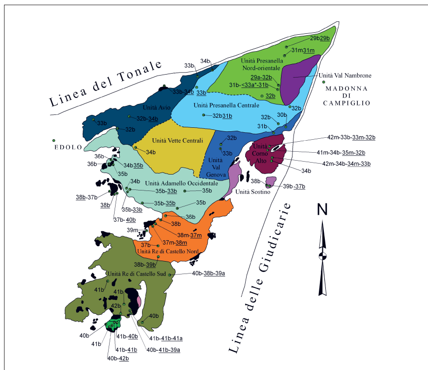
Fig. 2 – Schema geologico del batolite dell'Adamello e dati cronologici (da MACERA et alii , 1985). Abbreviazioni: (m) e (b) = età sulla muscovite e biotite con metodo Rb/Sr; ( m ) e ( b ) = età sulla muscovite e biotite con metodo K/Ar; (a) = età sull'orneblenda con metodo k/Ar; ( a *) = età sull'orneblenda con metodo ^{40}\text{Ar}/^{39}\text{Ar} . In nero le masse femiche.
