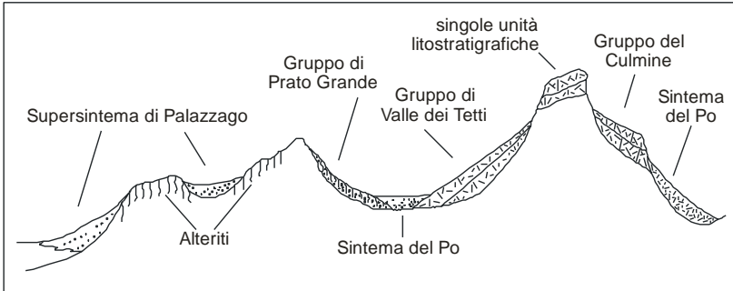
Fig.12 - Schema dei rapporti stratigrafici dei depositi di versante al raccordo versanti-pianura e in media valle.
