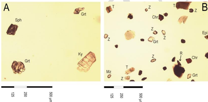
Fig. 12 – Suites a minerali pesanti della successione cretacea nell’area di studio. A = F.ne di Sorisole (Valle del Gatton): petrofacies a dominante cristallina, con cianite (Ky), granato (Grt) e titanite (Sph). B = flysch di Pontida (Isella): petrofacies a dominante sedimentaria e vulcanica, con zirconio (Z), tormalina (T), rutilo (R), cromopicitite (Chr), epidoto (Epi), granato (Grt) e monazite (Mz). Foto in luce polarizzata trasmessa, nicol paralleli.
