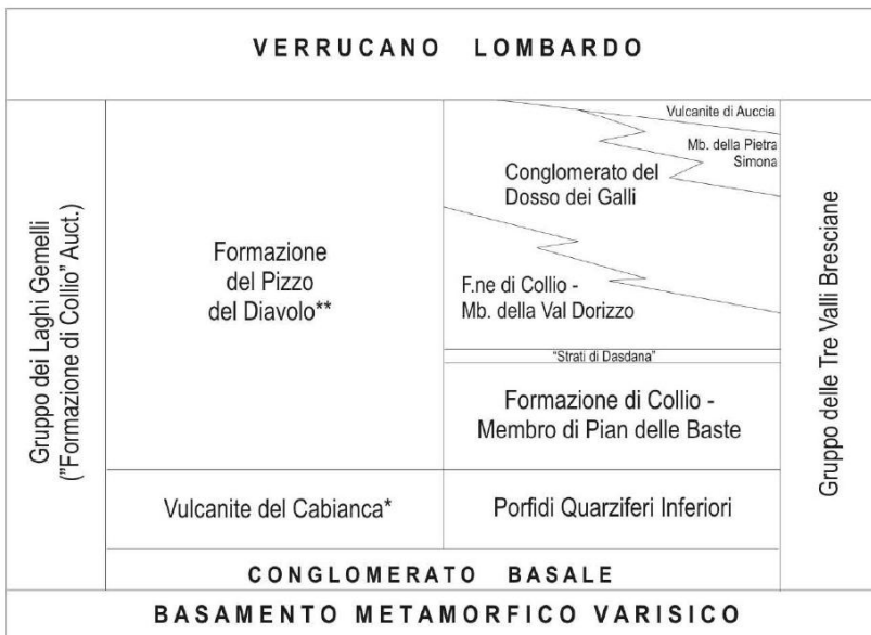
Fig. 4 – Revisione nomenclaturale della successione di età Permiano inferiore in Lombardia
