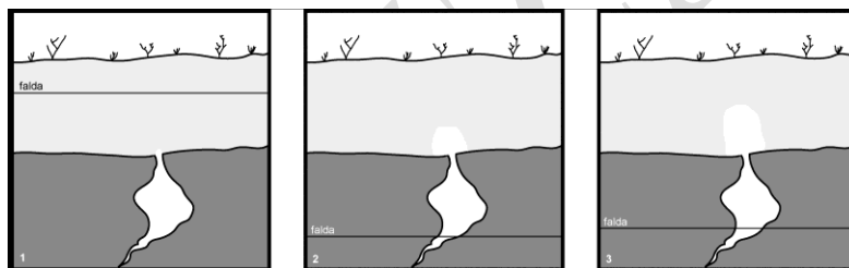
Fig. 14 - Meccanismo di innesco e sviluppo nel caso di cavità in terreni legate alla presenza di conglomerato. Nella situazione iniziale (1) si ha un conglomerato sottostante (grigio scuro) con cavità carsiche o fratture allargate che funge da livello permeabile, coperto da sedimenti alterati poco permeabili (grigio chiaro). Quando la falda si abbassa (2) si generano fenomeni di piping al contatto tra i due sedimenti con formazione di piccole cavità. Una volta formatasi, la cavità si evolve (3) per piping in occasione di ogni successiva venuta d'acqua e per crolli successivi.
