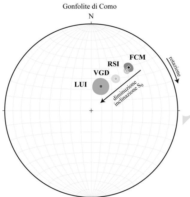
Fig. 11 – Proiezione stereografica equiareale (emisfero inferiore) del valore medio e del cono di confidenza ( \alpha_{95} ) dei poli delle giaciture S_0 per ciascuna unità della Gonfolite di Como. La direzione e l'inclinazione delle S_0 variano progressivamente dalle peliti di Prestino (RSI) ai conglomerati di Lucino (LUI).
