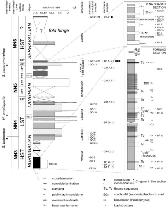
Fig. 8 - Sezione schematica della Gonfolite nel Settore della Brianza (da: SCIUNNACH & TREMOLADA, 2004).
