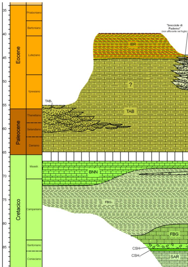
Fig. 3 – Schema crono-litostratigrafico delle unità cretaceo-eoceniche.
