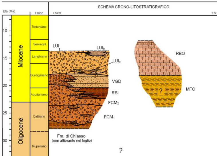
Fig. 6 – Schema cronolitostratigrafico delle unità oligo-mioceniche.
