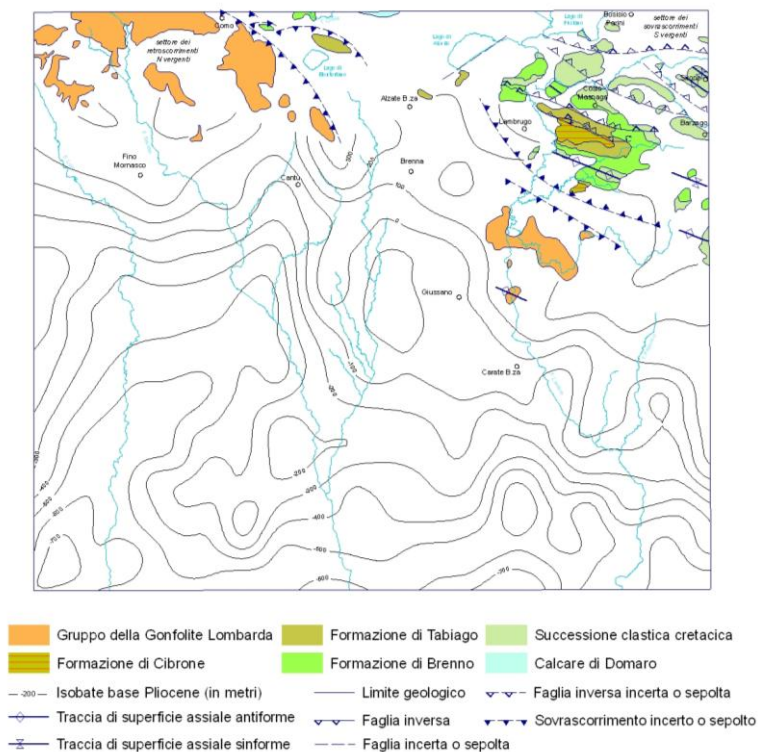
Fig. 9 - Schema strutturale del Foglio 096 - Seregno.
