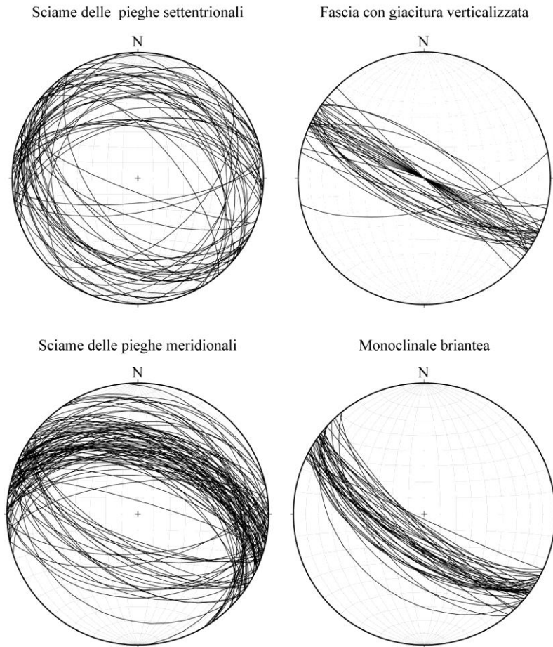
Fig. 10 – Proiezione stereografica equiareale (emisfero inferiore) delle giaciture S_0 misurate nel Settore dei sovrascorrimenti S-vergenti.
