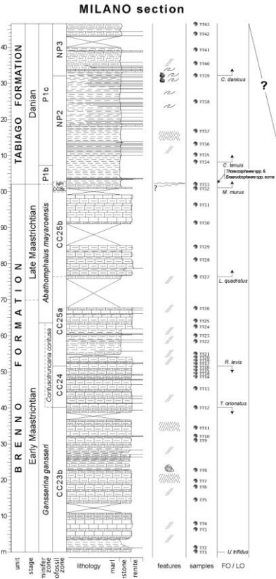
Fig. 4 - Sezione stratigrafica della formazione di Tabiago lungo la SS. 36.
