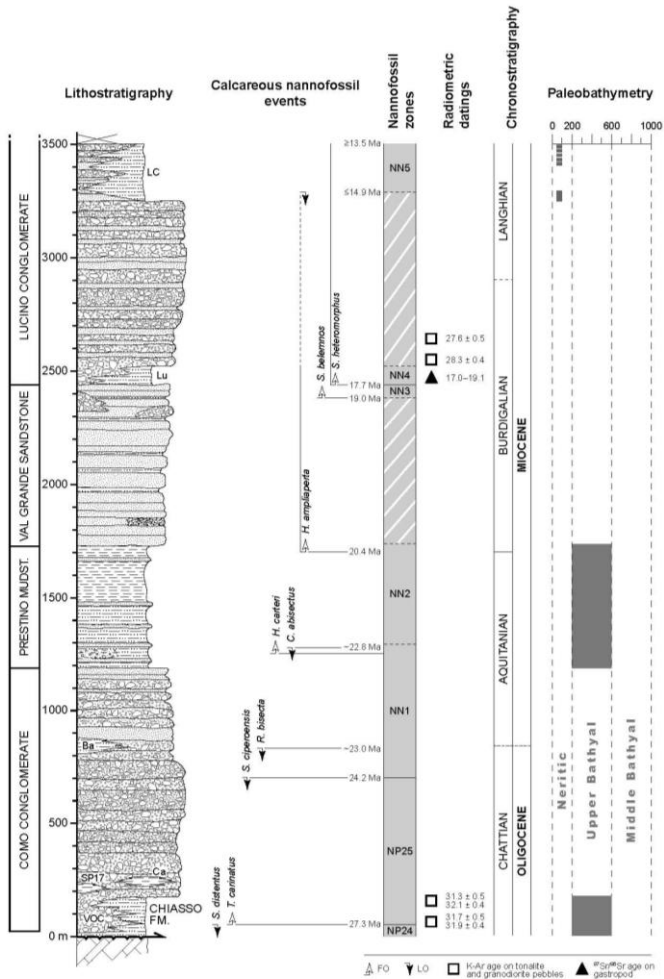
Fig. 7 - Sezione schematica della Gonfolite nel Settore di Como.
