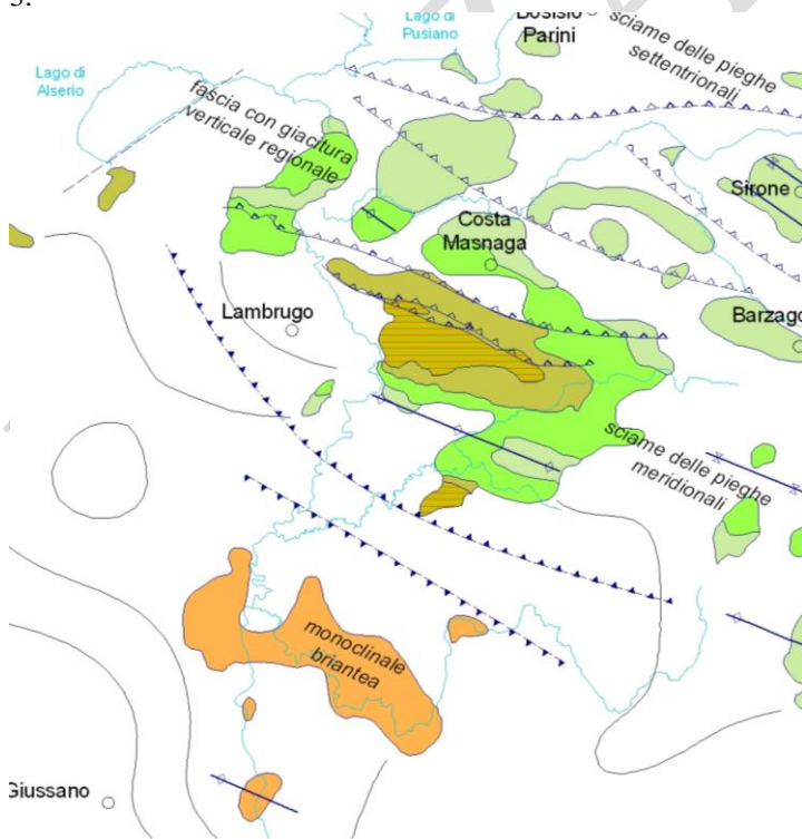
Fig. 9a - Dettaglio del settore NE del foglio (Settore dei spovrascorimenti S - vergenti).
