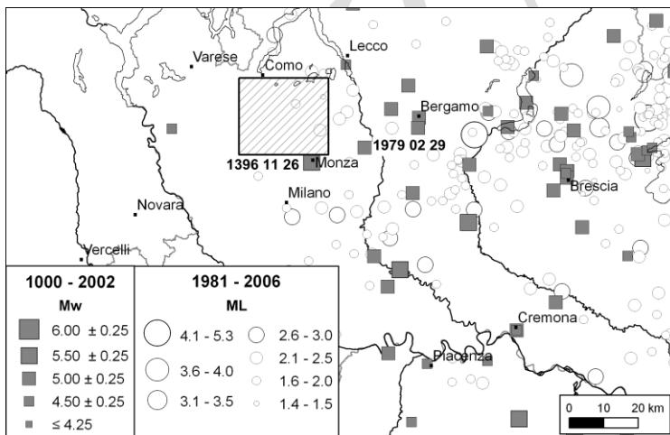
Fig. 12 - Sismicità 1000-2002 da CPTI04 (Gruppo di lavoro CPTI, 2004) e 1981-2006 da CSI 1.1 (CASTELLO et alii , 2006 e Bollettino Strumentale INGV). (Mw= magnitudo momento, ML=magnitudo locale).
