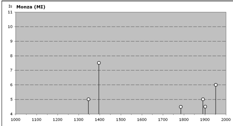
Fig. 13 - Grafico della storia sismica di Monza, da DBMI04 (STUCCHI et alii, 2007). (Is = Intensità al sito (MCS)).
