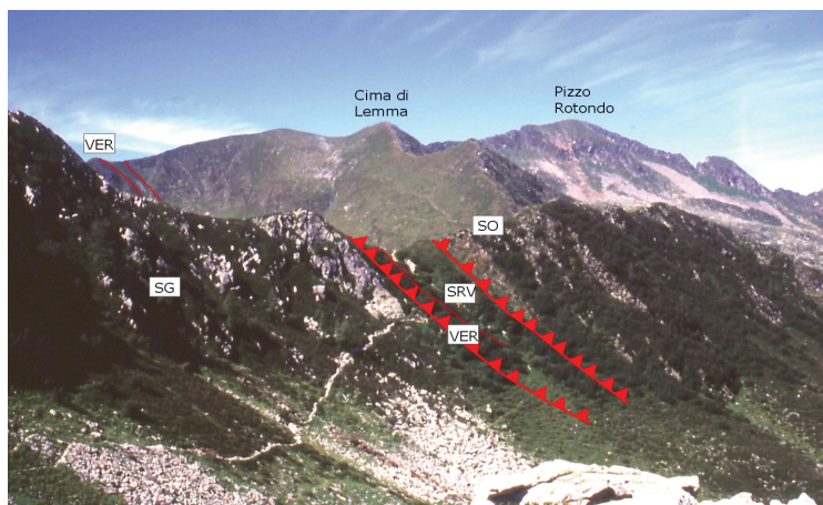
Fig. 26 - Lembi sedimentari di Servino (SRV) e Verrucano Lombardo (VER) implicati lungo la Linea del Porcile, tra Settore Orobico (SO) e Settore della Gallinera (SG) – Passo Tartano. La foto è ripresa da NE.
