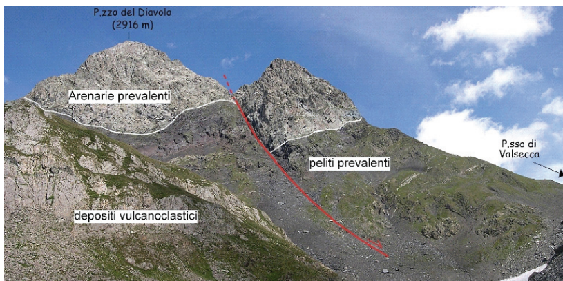
Fig. 16 - Sedimenti continentali alluvio-lacustri del Permiano inferiore presso il Pizzo del Diavolo e il "Diavolino" (appartenenti all'omonima formazione). Da SW verso NE (alta Val Camisana).
