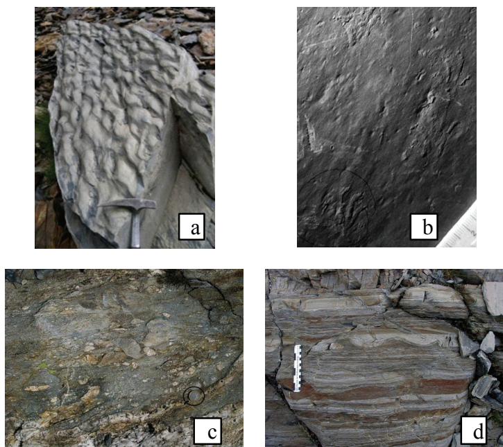
Fig. 17 – a) Ripples linguoidi nei depositi lacustri permiani in prossimità del Passo di Valsecca; b) Impronte di Dromopus lacertoides , tetrapodi del Permiano inferiore (Foto G. Santi, Passo di Valsecca); c) depositi vulcanoclastici appartenenti alle vulcaniti intercalate nella formazione di Pizzo del Diavolo; d) Deformazioni da carico o sismite nei sedimenti fini laminati della formazione di Pizzo del Diavolo (Permiano inferiore)
