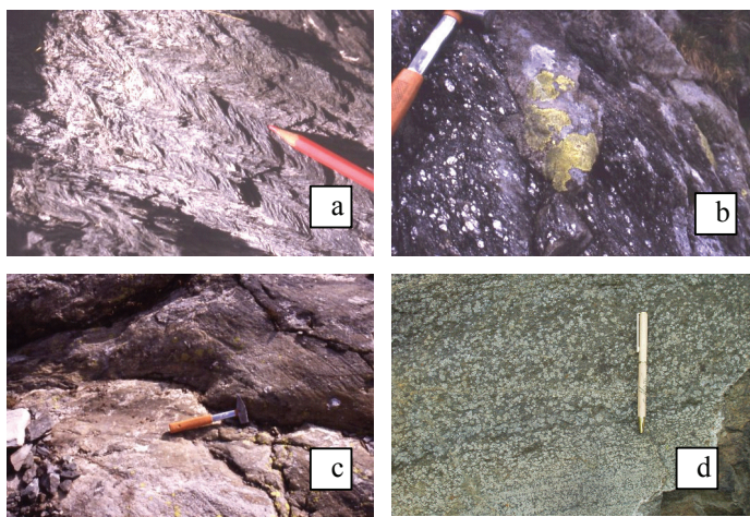
Fig. 12 – a) Filloniti - Evidente foliazione di crenulazione S_2 – Scale di Venina, Val Venina; b) Gneiss del Pizzo Meriggio – PRG. Tipica struttura occhiadina – Valle dei Lupi, alta Val Tartano; c) Contatto stratigrafico tra Gneiss di Morbegno – MOB, e conglomerati del gruppo dei Laghi Gemelli - LG – Passo del Forcellino, alta Val d'Ambria; d) Tipico aspetto degli Gneiss di Morbegno con "noduli" (peciloblasti) di oligoclasio, fino a 1 cm di diametro. Strada per Tartano q. 1000 m s.l.m.
