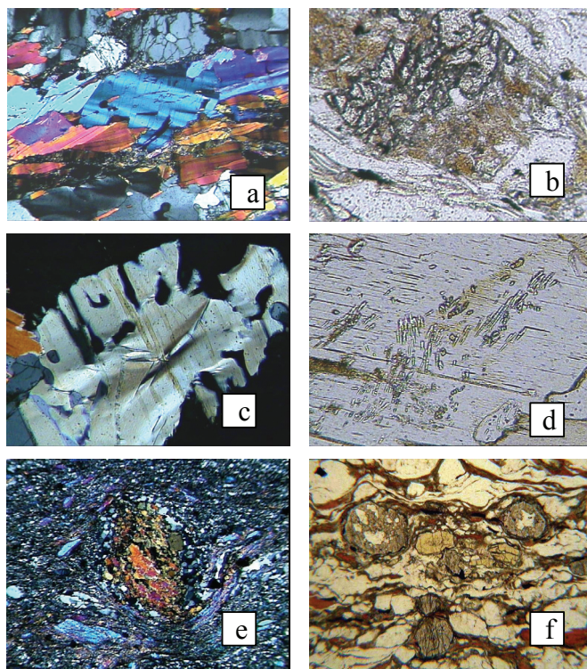
Fig. 5 - Unità degli Gneiss del Monte Tonale – Microfotografie di sezioni sottili: a) Paragneiss kinzigitico . Pol+, 15X - Muscovite cross deformata con relitti di sillimanite. Lungo la strada in sinistra idrografica del Torrente Davaglione, in prossimità di Alpe Arcino (q. 1675 m s.l.m.); b) Protomylonite di paragneiss Pol+, 15X - Granato parzialmente cloritizzato. Dalla clorite si forma biotite nuova. Lungo la strada a Nord di Postalesio in sinistra idrografica del Torrente Caldenno (q. 1000 m s.l.m.); c) Paragneiss kinzigitico Pol+, 15X - Muscovite cross deformata con gocce di quarzo (tipo mirmechite). Lungo la strada in sinistra idrografica Torrente Davaglione, in prossimità di Alpe Arcino (q. 1675 m s.l.m.); d) Paragneiss kinzigitico . Pol+, 20X - Muscovite cross deformata con inclusi di sillimanite relitta. Lungo la strada in sinistra idrografica Torrente Davaglione, in prossimità di Alpe Arcino (q. 1675 m s.l.m.); e) Milonite di paragneiss . Pol+, 10X - Porfiroclasto di tormalina ricristallizzato. Lungo la strada nel tratto tra Prasomaso e Premachera (q. 1330 m s.l.m.); f) Milonite di mica-schisto a Bt+Grt+St . Solo pol. 10X. - Lungo la strada in destra idrografica della Val Fontana, a nord delle Baite della Piana (q. 830 m s.l.m.).
