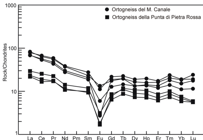
Fig. 4 - Pattern delle REE, normalizzato alla condrite CI (NAKAMURA, 1974) degli ortogneiss occhiadini a due miche appartenenti all'unità degli Gneiss della Punta di Pietra Rossa (Austroalpino superiore) e degli ortogneiss del Monte Canale (Austroalpino inferiore) (BERGOMI et alii, 2005).
