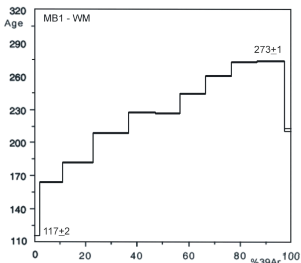
Fig. 25 - Spettro di età apparente Ar/Ar su WM appartenente ad un campione di Gneiss Chiari del Corno Stella milonitico campionato lungo la Linea del Porcile (BERGOMI, 2004)
