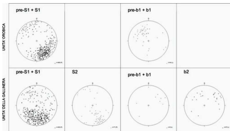
Fig. 28 - Diagrammi equiareali di Schmidt nei quali sono riportate le foliazioni (S) e le lineazioni (b) prealpine del basamento metamorfico sudalpino.
