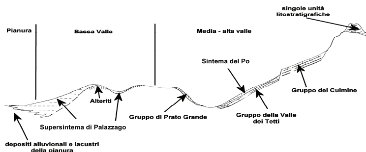
Fig. 20 - Schema dei rapporti stratigrafici dei depositi di versante, al raccordo tra versanti e pianura e in media valle.
