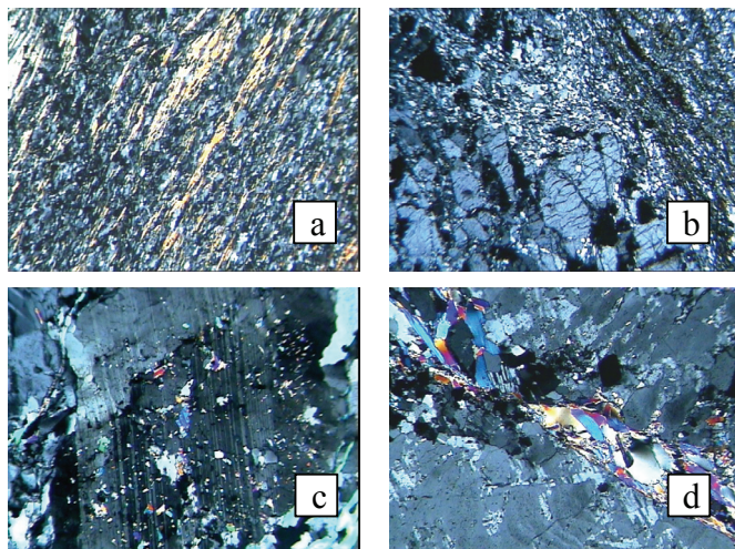
Fig. 3 – Unità degli Gneiss della Punta di Pietra Rossa - Microfotografie di sezioni sottili: a) Mylonite di gneiss minuto . Pol+, 10X - Lungo la strada per Sasso, sopra Triangia, nel tratto tra Prasomaso e Premachera (q. 1370m s.l.m.); b) Mylonite di ortogneiss occhiadino a due miche . Pol+, 15X - Porfiroclasto feldspatico. Val Fontana. c) Ortogneiss occhiadino a due miche . Pol+, 15X - Plagioclasio con zonatura ignea conservata. Lungo la strada a Nord di Regoledo, nel tratto Sogno-Prà Balzar (q. 980 m s.l.m.); d) Ortogneiss occhiadino a due miche . Pol+, 15X - K-feldspato concresciuto con plagioclasio. Lungo la strada a Nord di Regoledo, nel tratto Sogno-Prà Balzar (q. 980 m s.l.m.).
