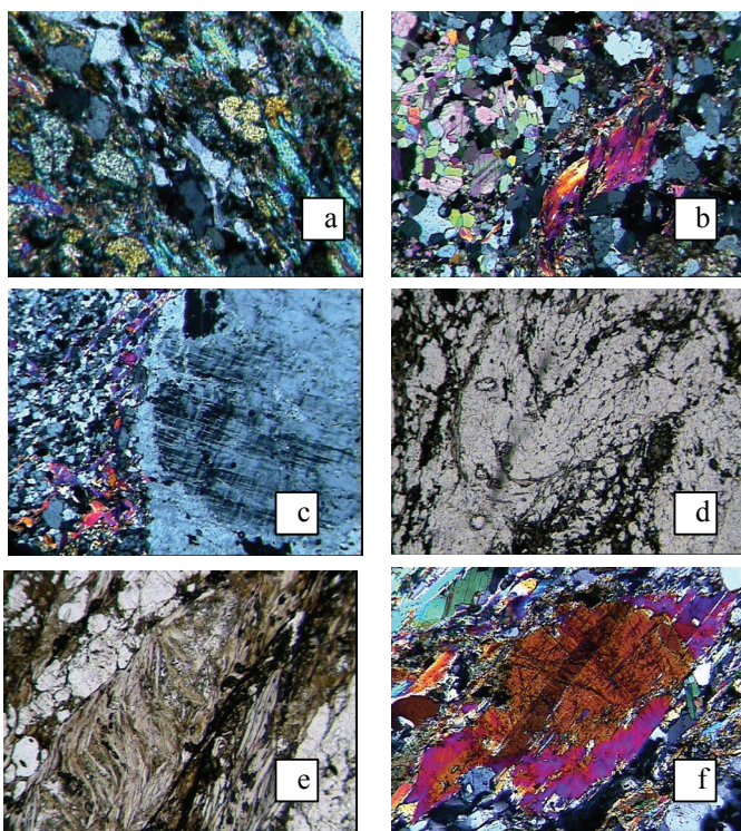
Fig. 2 - Unità degli Gneiss del Monte Canale - Microfotografie di sezioni sottili: a) Paragneiss ricco di epidoto, con Ab, Qtz, Bt, Cc. Pol+, 10X. A Nord di Prà Isio, lungo la mulattiera (q. 1720 m s.l.m.) verso Alpe Caldenno; b) Calcescisto. Pol+, 10X - Cc, Chl, Qtz, Ab e mica chiara verdina. A Nord di Prà Isio, lungo la mulattiera (q. 1685 m s.l.m.) verso Alpe Caldenno; c) Ortogneiss. Pol+, 15X - Ortogneiss derivato da una facies porfirica del protolite granitico - porfiroclasto di microclino con bordo di plagioclasio mirmechitico. A Nord di Prà Isio, lungo mulattiera (q. 1710 m s.l.m.) verso Alpe Caldenno; d) Milonite di ortogneiss con pieghe. Solo pol. 10X - Località Prati, lungo il sentiero in destra idrografica del Torrente Caldenno (q. 1380 m s.l.m.); e) Paragneiss incassante dell'ortogneiss. Solo pol. 10X - Struttura SC nelle bande a clorite che si trasforma in biotite, a Nord di Prà Isio lungo la mulattiera (q. 1730 m s.l.m.) verso Alpe Caldenno; f) Ortogneiss. Pol+, 15X - Anfibolo zonato. Il nucleo (reliitto magmatico) è composto di orneblenda, il bordo è attinolitico. Sopra Prà Curati, strada Torre Santa Maria - La Foppaccia (q. 1300 m s.l.m.).
