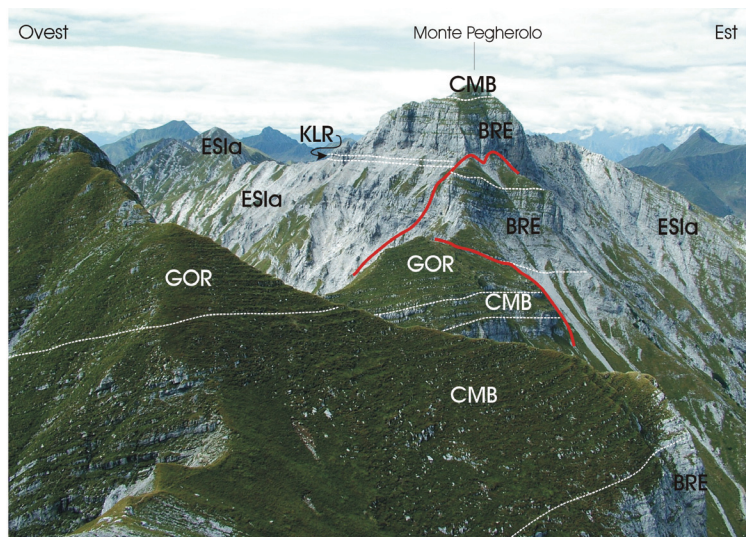
Fig. 19: Panorama del Monte Pegherolo da sud. È evidente il passaggio tra le facies massicce e clinostatificate del calcare di Esino ( ESla ) e la soprapostante successione carnica a stratificazione orizzontale costituita da Formazione di Breno (BRE), Calcare Metallifero Bergamasco (CMB) e formazione di Gorno (GOR). Tra ESla e BRE è presente un sottile livello con breccie ed evidenze di emersione che corrisponde al calcare Rosso (KLR). La presenza di faglie normali (linee rosse) abbassa il settore del Monte Secco rispetto alla cima del Monte Pegherolo.
