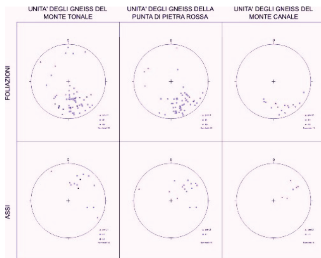
Fig.24 - Diagrammi equiareali di Schmidt nei quali sono riportate le strutture prealpine delle unità austroalpine
