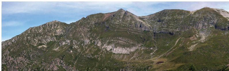
Fig. 14 - Panorama Monte Masoni (alta valle del Fiume Brembo visto da SSE). Lungo le pendici Sud-orientali si osservano, oltre al Conglomerato Basale, una litofacies della Vulcanite del Cabianca e le litofacies sedimentarie della formazione del Pizzo del Diavolo.
