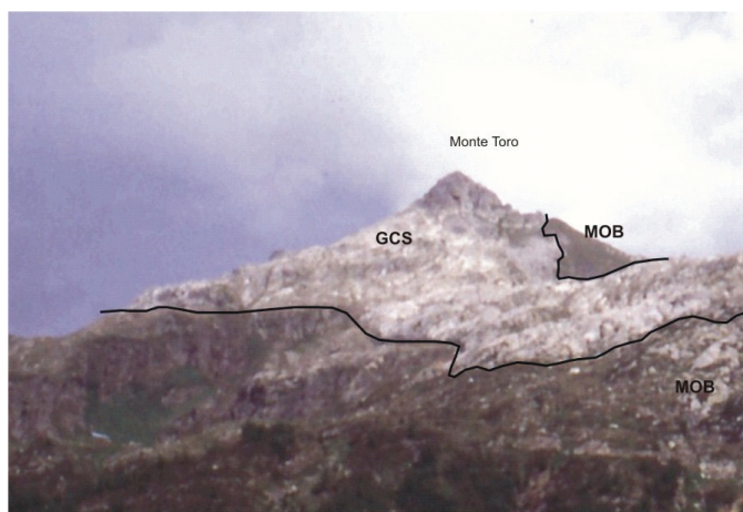
Fig. 11 - Contatto tra Gneiss Chiari del Corno Stella (GCS) e Gneiss di Morbegno (MOB) visto da NW. Versante NE del Monte Toro.
