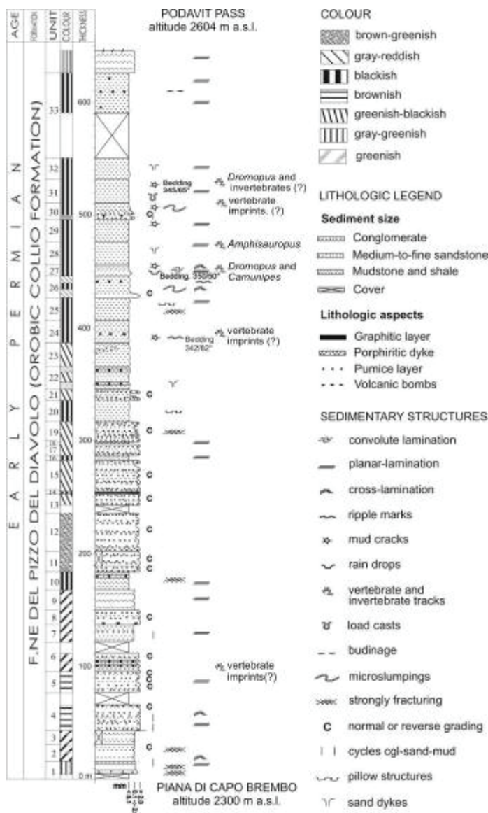
Fig. 15 - Sezione stratigrafica delle unità vulcanoclastiche e sedimentarie alluvio-lacustri (membro sedimentario della Formazione di Collio = formazione di Pizzo del Diavolo) misurata nell'area del Pizzo del Diavolo (RONCHI et alii, 2005).
