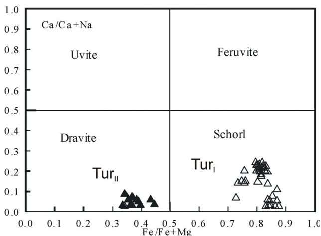
Fig. 10 - Diagramma composizionale delle tormaline provenienti dagli Gneiss Chiari del Corno Stella (BERGOMI, 2004 a ).
