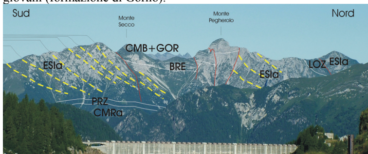
Fig. 18: Panorama del Monte Pegherolo da est (rifugio Calvi). Nella figura si nota la successione triassica dal Calcare di Camorelli (CMR a ) fino alla formazione di Gorno che costituisce la cima del Monte Secco, ribassato da alcune faglie normali rispetto alla cima
